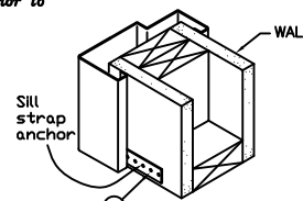
OPTIONAL SILL ANCHOR
