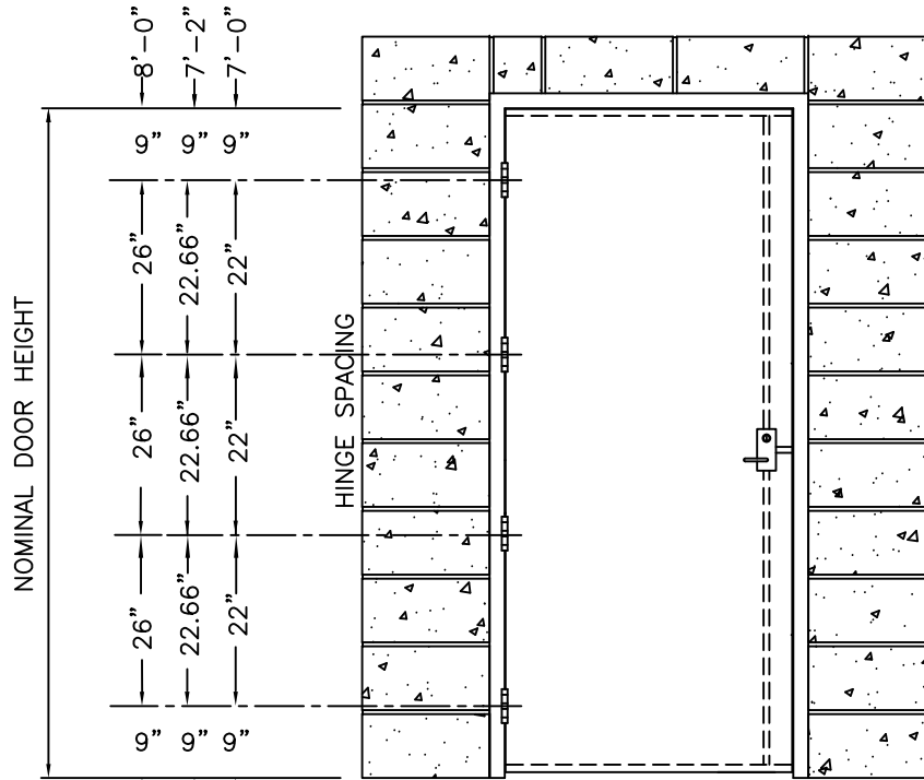
ELEVATION
