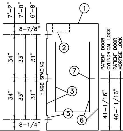
DOOR ELEVATION
