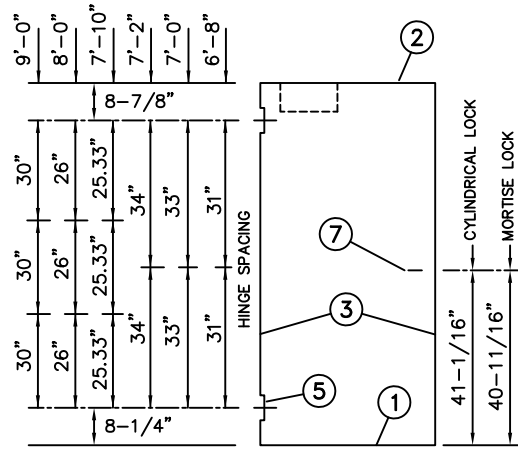
DOOR ELEVATION
